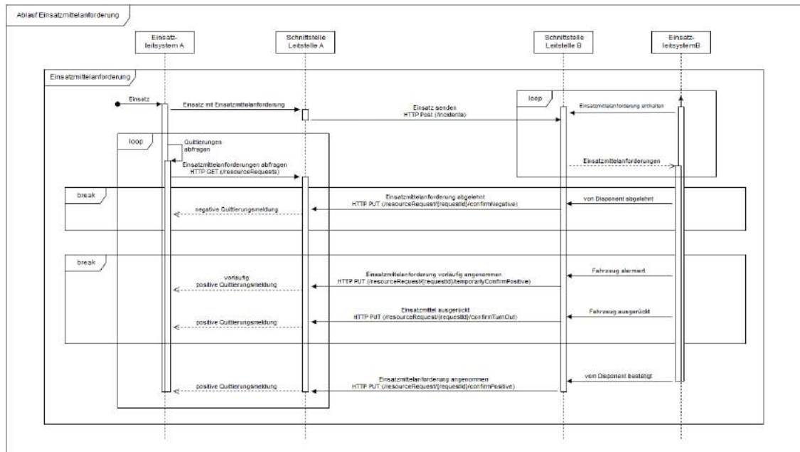
Abbildung 3: Ablauf Einsatzmittelanforderung
