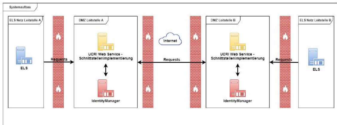
Abbildung 1: Systemaufbau
