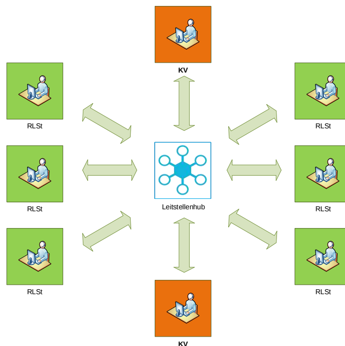
Abbildung 3: Kommunikationsarchitektur mit Leitstellenhub
