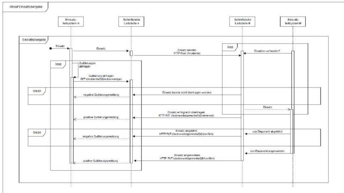
Abbildung 2: Ablauf Einsatzübergabe
